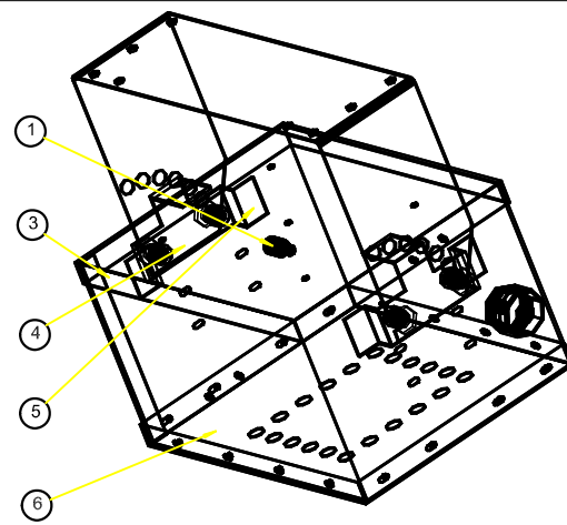
Iso View(Bottom)
